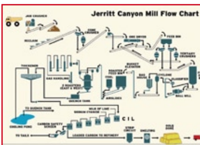
Jerritt Canyon Nevada Ablauf Golderzverarbeitung
